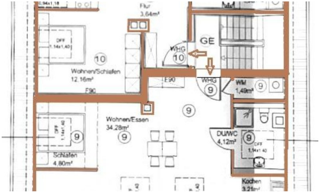
Grundrissplan-Dachspeicher (Grundriss)
